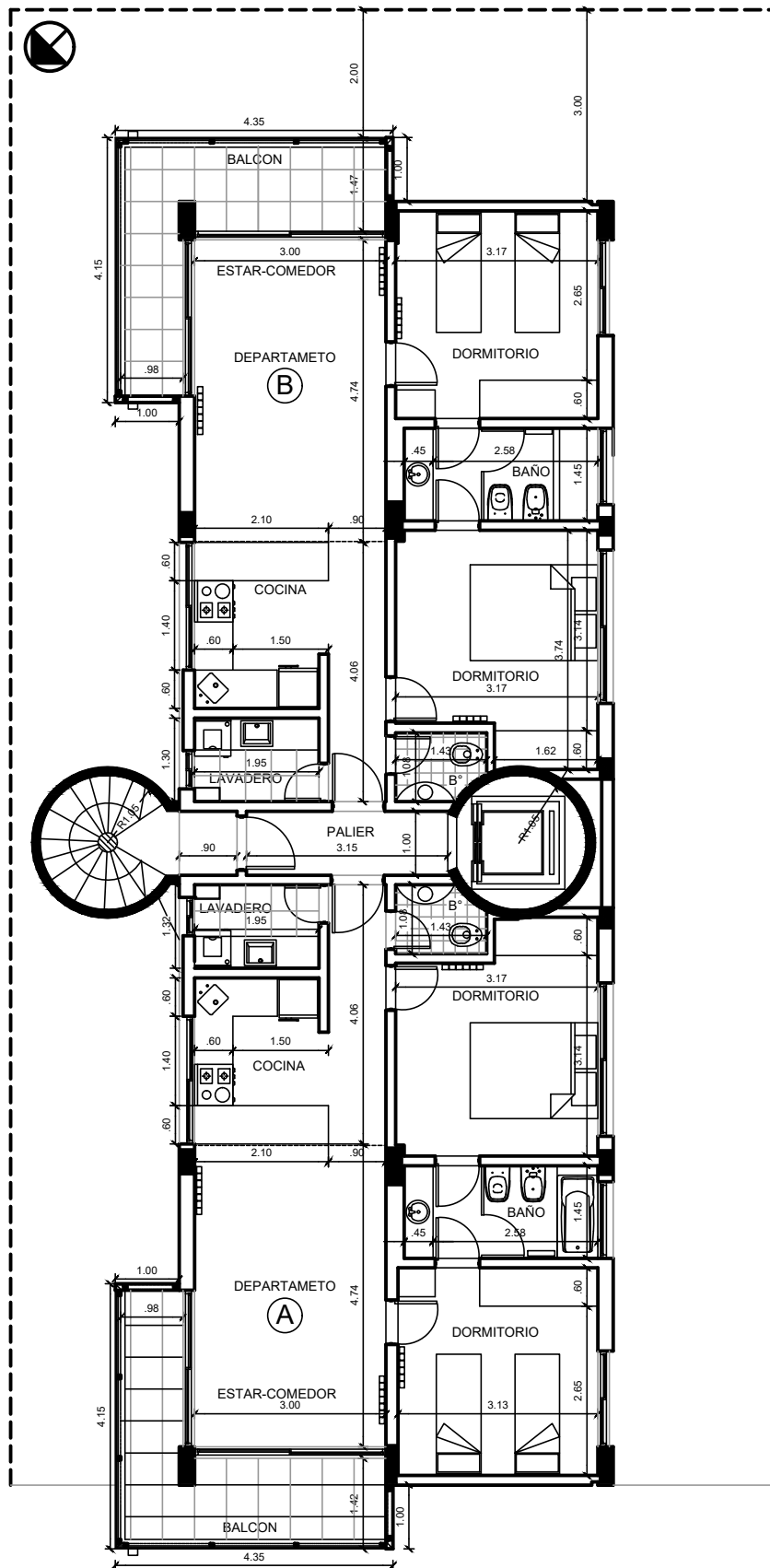
PLANTA TIPO 1er. al 5to.PISO NIVEL +3.00 a +15.00m
