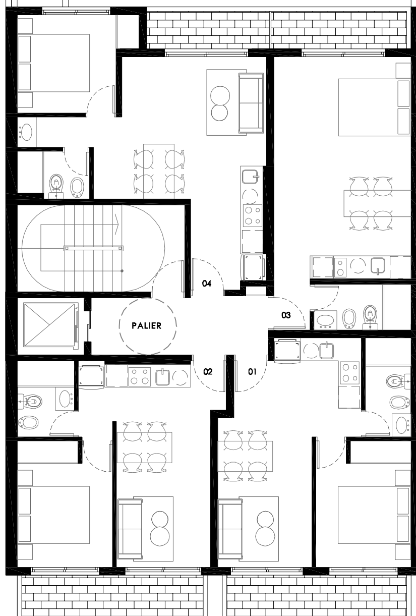
PLANTA TIPO DEL 1 AL 8
